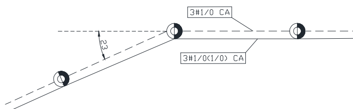
Figura 1 – Resultante de tração mecânica com dois esforços
